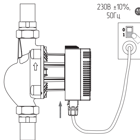
Рис. 36 Электроподключение насоса
